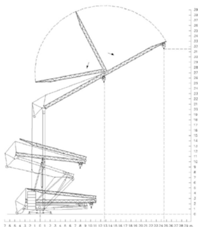
PLUMA INCLINADA 30°
